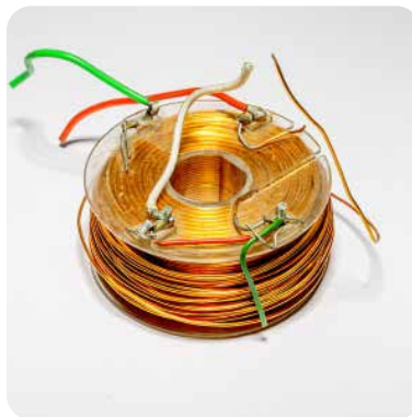
Kupferspule
